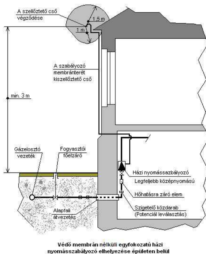
b) Épületen belül középnyomású házi nyomásszabályozó
